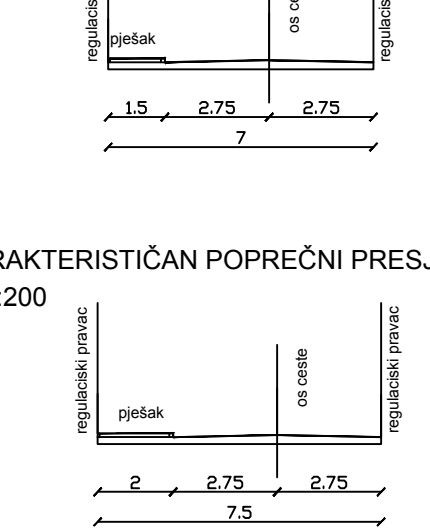
KARAKTERISTIČAN POPREČNI PRESJEK A - A M 1:200
